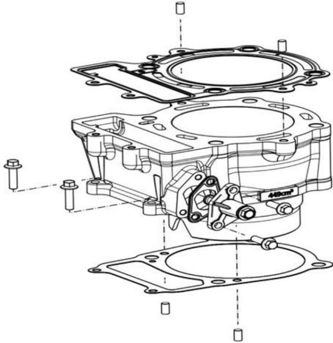
气缸体部件 CYLINDER ASSEMBLY
