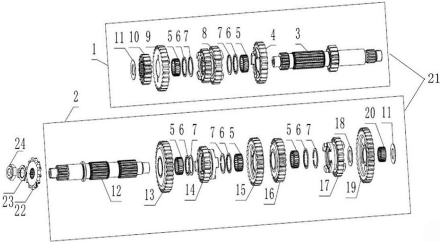
主副轴组合 TRANSMISSION MAIN,COUNTER SHAFT
