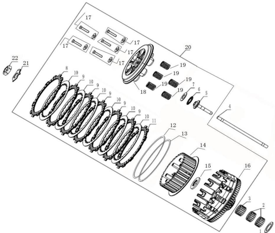
离合器总成 CLUTCH ASSY
