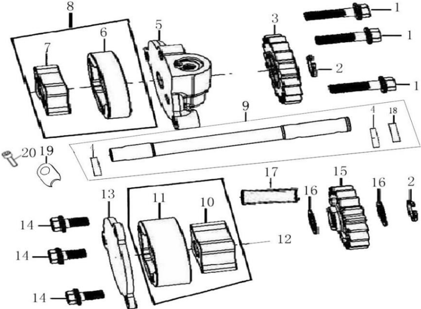
机油泵部件 OIL PUMP
