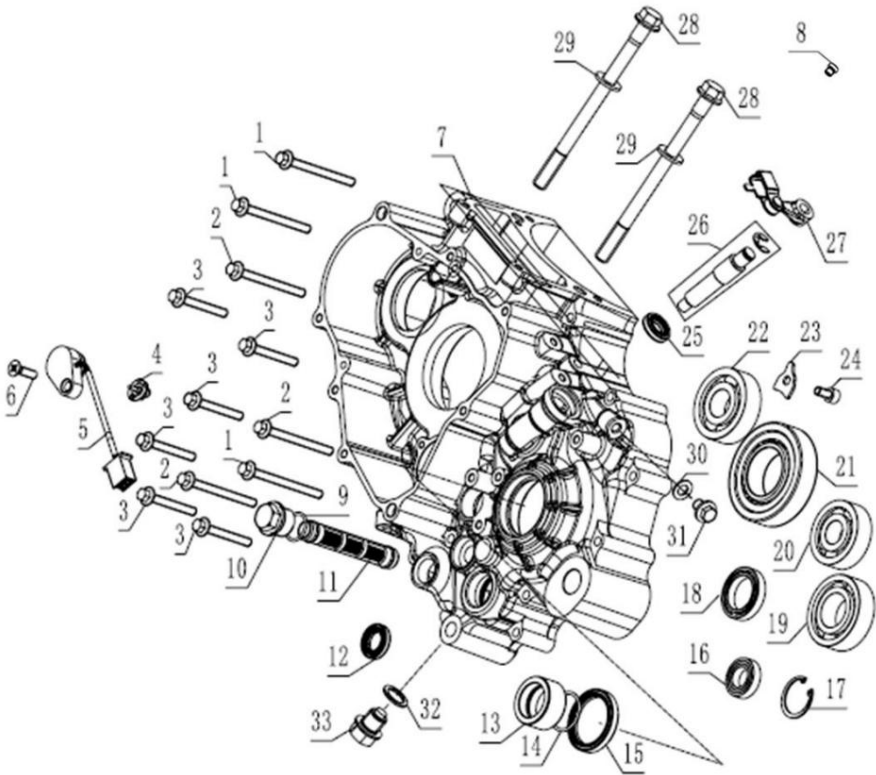
左曲轴箱 LEFT CRANKCASE
